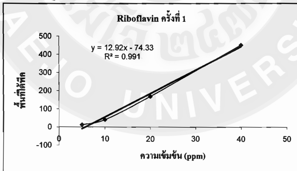
ภาพที่ 9 กราฟมาตรฐานไรโบฟลาวิน ครั้งที่ 1 (วัดค่าการดูดกลืนแสง 280 นาโนเมตร)
