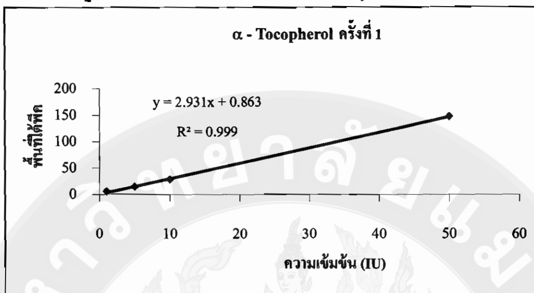
ภาพที่ 3 กราฟมาตรฐานแอลฟา-โทโคฟีรอล ครั้งที่ 1 (วัดค่าการดูดกลืนแสง 335 นาโนเมตร)
