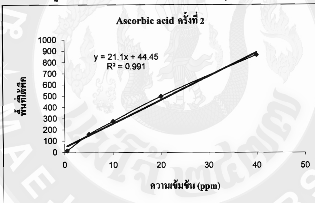
ภาพที่ 6 กราฟมาตรฐานกรดแอสคอร์บิก ครั้งที่ 2 (วัดค่าการดูดกลืนแสง 244 นาโนเมตร)
