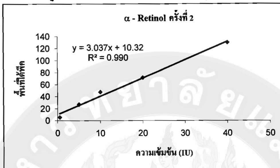
ภาพที่ 2 กราฟมาตรฐานแอลฟา-เรตินอล ครั้งที่ 2 (วัดค่าการดูดกลืนแสง 335 นาโนเมตร)
