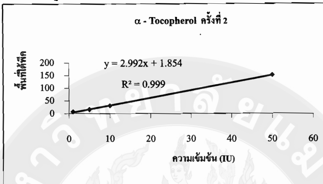
ภาพที่ 4 กราฟมาตรฐานแอลฟา-โทโคฟีรอล ครั้งที่ 2 (วัดค่าการดูดกลืนแสง 335 นาโนเมตร)
