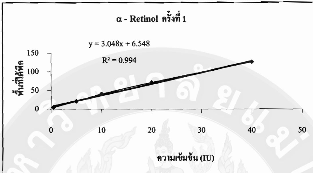
ภาพที่ 1 กราฟมาตรฐานแอลฟา-เรตินอล ครั้งที่ 1 (วัดค่าการดูดกลืนแสง 335 นาโนเมตร)
