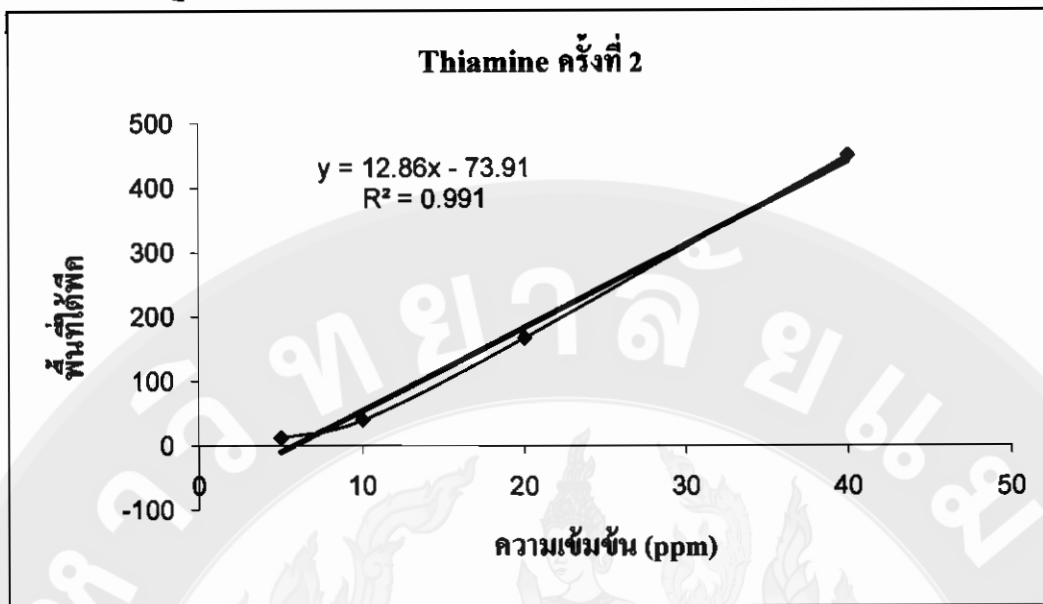
ภาพที่ 8 กราฟมาตรฐานไทอามีน ครั้งที่ 2 (วัดค่าการดูดกลืนแสง 280 นาโนเมตร)
