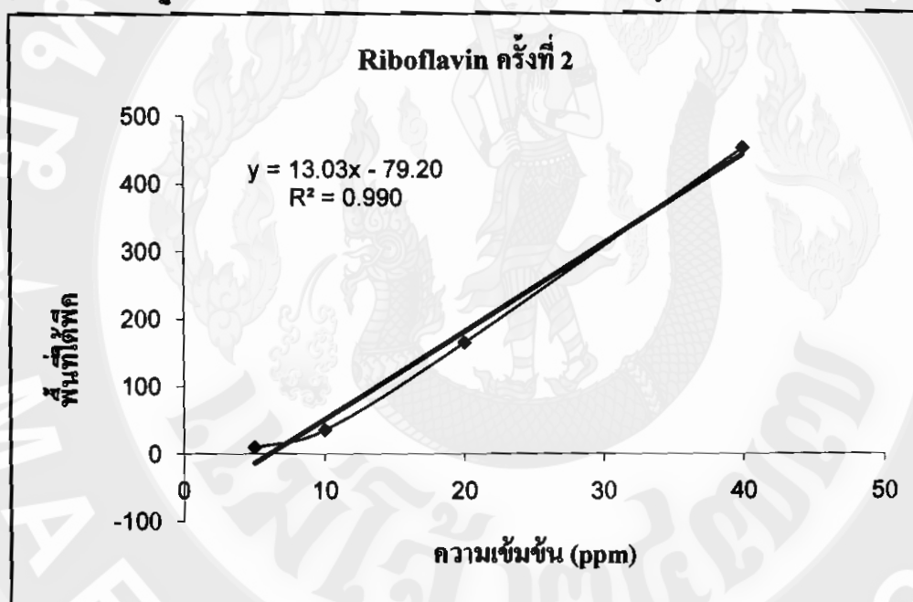
ภาพที่ 10 กราฟมาตรฐานไรโบฟลาวิน ครั้งที่ 2 (วัดค่าการดูดกลืนแสง 280 นาโนเมตร)
